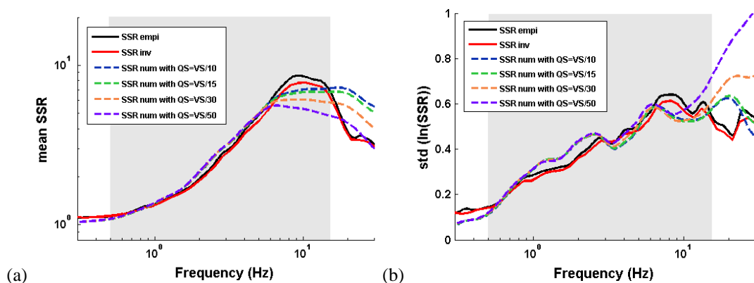
Figure 6. (a) Comparaison des moyennes globales des rapports spectraux et (b) les écarts-types associés obtenus à partir de l'approche empirique (en noir), de l'inversion généralisée (en rouge) et des simulations numériques (lignes discontinues).
