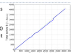
Fig. 5.a : le chemin optimal obtenu par IDDTW
