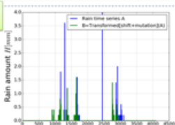
Fig. 4 : la série d'origine + la série transformée
