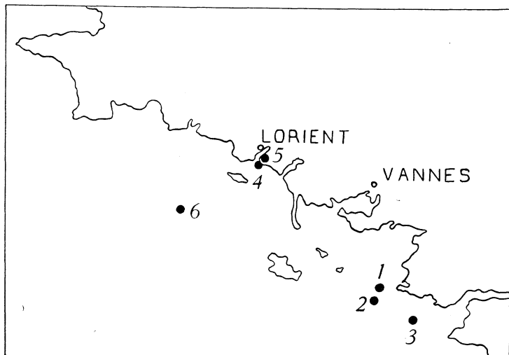
FIG. 1. — Gisements de Nummulites des côtes méridionales de Bretagne. — 1, plateau du Four ; 2, banc de Guérande ; 3, rochers de la Banche ; 4, pointe de Gâvre ; 5, tranchée de Locmalo ; 6, station 441, dragage du Président Théodore-Tissier .
