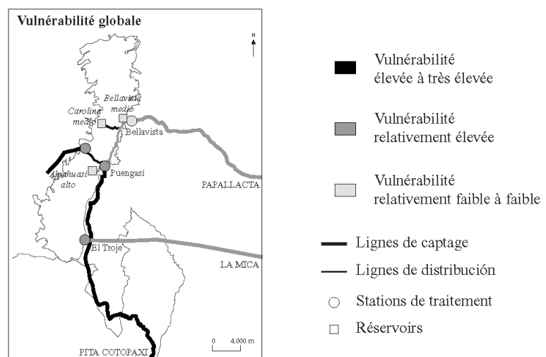
Carte 3 – Vulnérabilité des enjeux majeurs du système d'alimentation en eau potable du district métropolitain de Quito. Map 3 – Vulnerability of critical facilities for the water supply system in the Metropolitan District of Quito.
