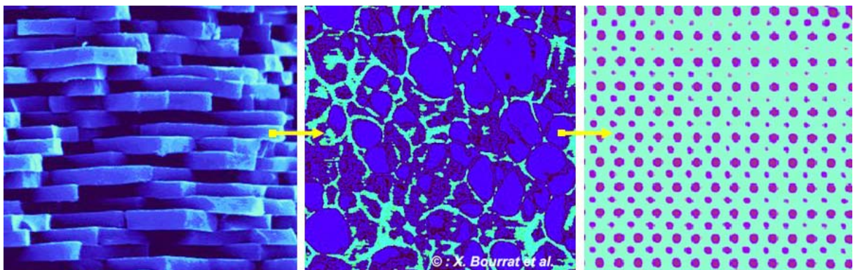
Figure 2. L'observation de la Nacre avec des grossissements croissant met en évidence sa structure multiéchelle : a) au microscope à balayage (MEB) ( 50 \times 50 \mu\text{m}^2 ) ; b) au microscope à force atomique (AFM) ( 0,5 \times 0,5 \mu\text{m}^2 ) ; c) au microscope électronique en transmission (MET) ( 0,005 \times 0,005 \mu\text{m}^2 )
