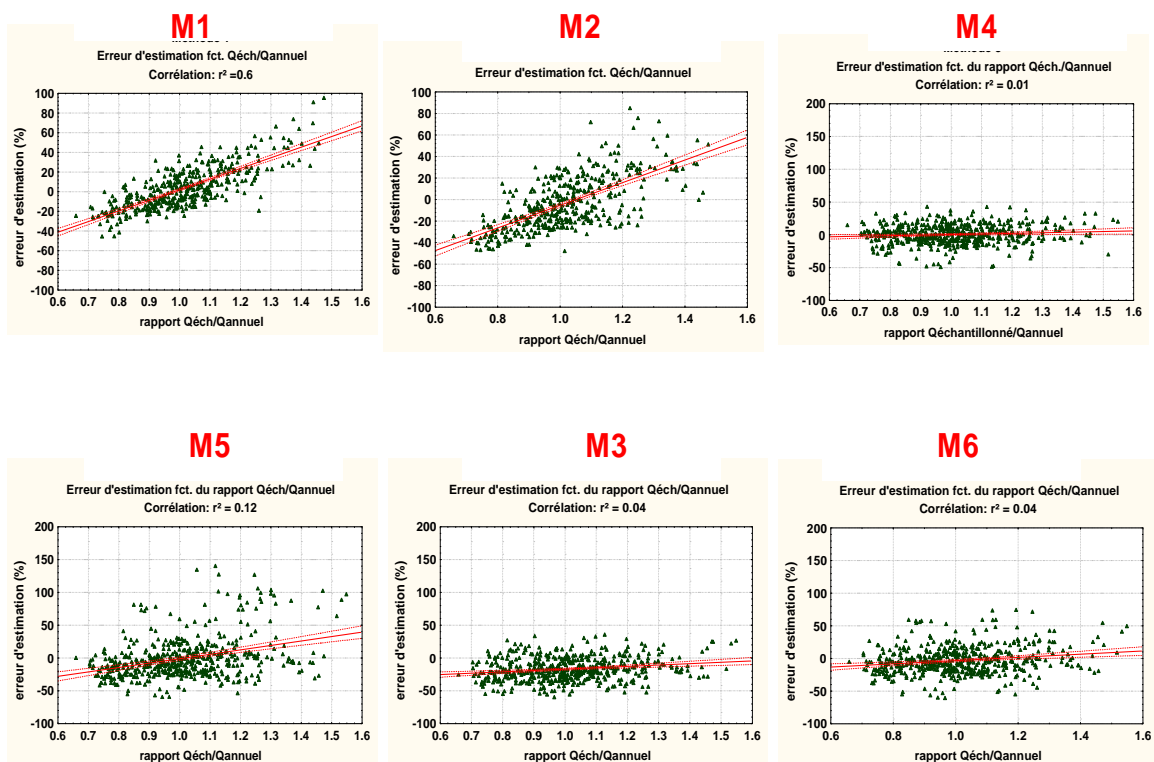
Figure 3. Erreurs sur les flux annuels en fonction du rapport des débits échantillonnés ( Q_{éch} ) au débit annuel \bar{Q} pour 6 méthodes de calcul des flux. La Loire à Orléans. Fréquence mensuelle.
