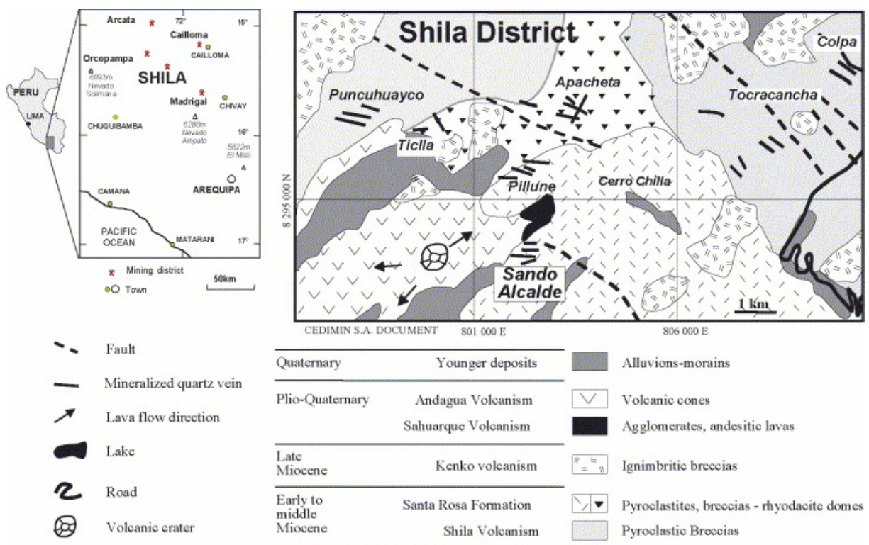
Fig. 1. Geological map of the Shila district. The location of the main deposits of the district is indicated (modified from a CEDIMIN SA document). Carte géologique du district de Shila. Les principaux gisements constituant ce district sont indiqués (modifié d'après un document Cedimin SA).
