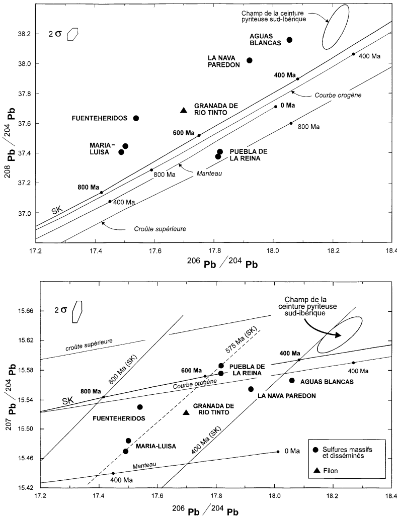
Figure 2. Compositions isotopiques du plomb des minéralisations analysées dans les diagrammes Pb/Pb. SK : courbe de croissance normale de Stacey–Kramers [17]; les autres courbes de croissance du plomb sont extraites de Doe et Zartman [5].
