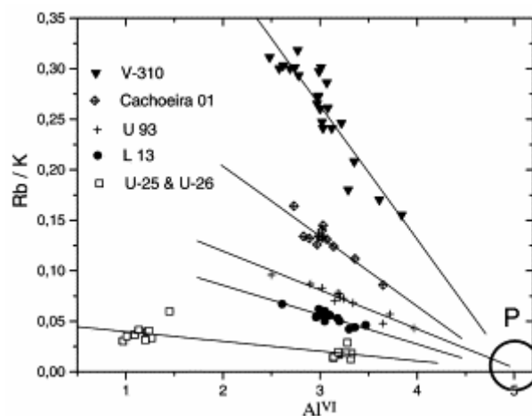
Fig. 1. Diagrammes [Rb/K] - [Al^{VI}] pour les micas des pegmatites : V310 , Volta Grande ; C01 , Cachoeira 01 ; U93 , Urubu, zone de contact ; L13 , José de Linto ; U25
