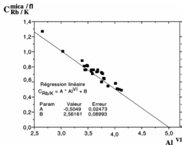
Fig. 2. C_{Rb/K}^{mica/fl} en fonction de [Al^{VI}] pour les micas des pegmatites de Volta Grande. Les points ont été obtenus en utilisant les valeurs mesurées [Rb/K] des feldspaths potassiques associés aux micas, connaissant le coefficient de partage expérimental de Rb entre feldspath et fluide. [Rb/K] versus [Al^{VI}] for micas from the Volta Grande pegmatites. Points were obtained using the [Rb/K] measured values of potash feldspars associated to micas, knowing the experimental partition coefficient of Rb between feldspar and fluid.
