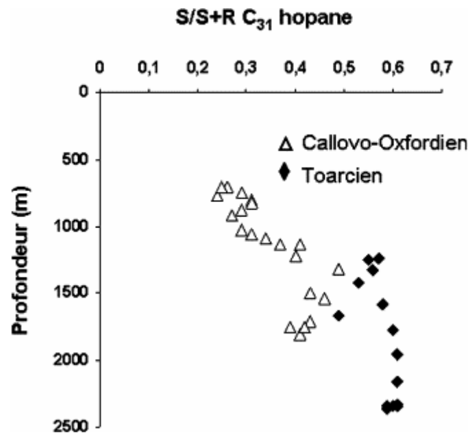
Fig. 3. Relation entre profondeur et rapports d'isomérisation S/R des C 31 hopane pour les différents puits considérés dans cette étude. - Relationship between depth and C 31 hopane S/R isomerisation ratios for the studied wells.
