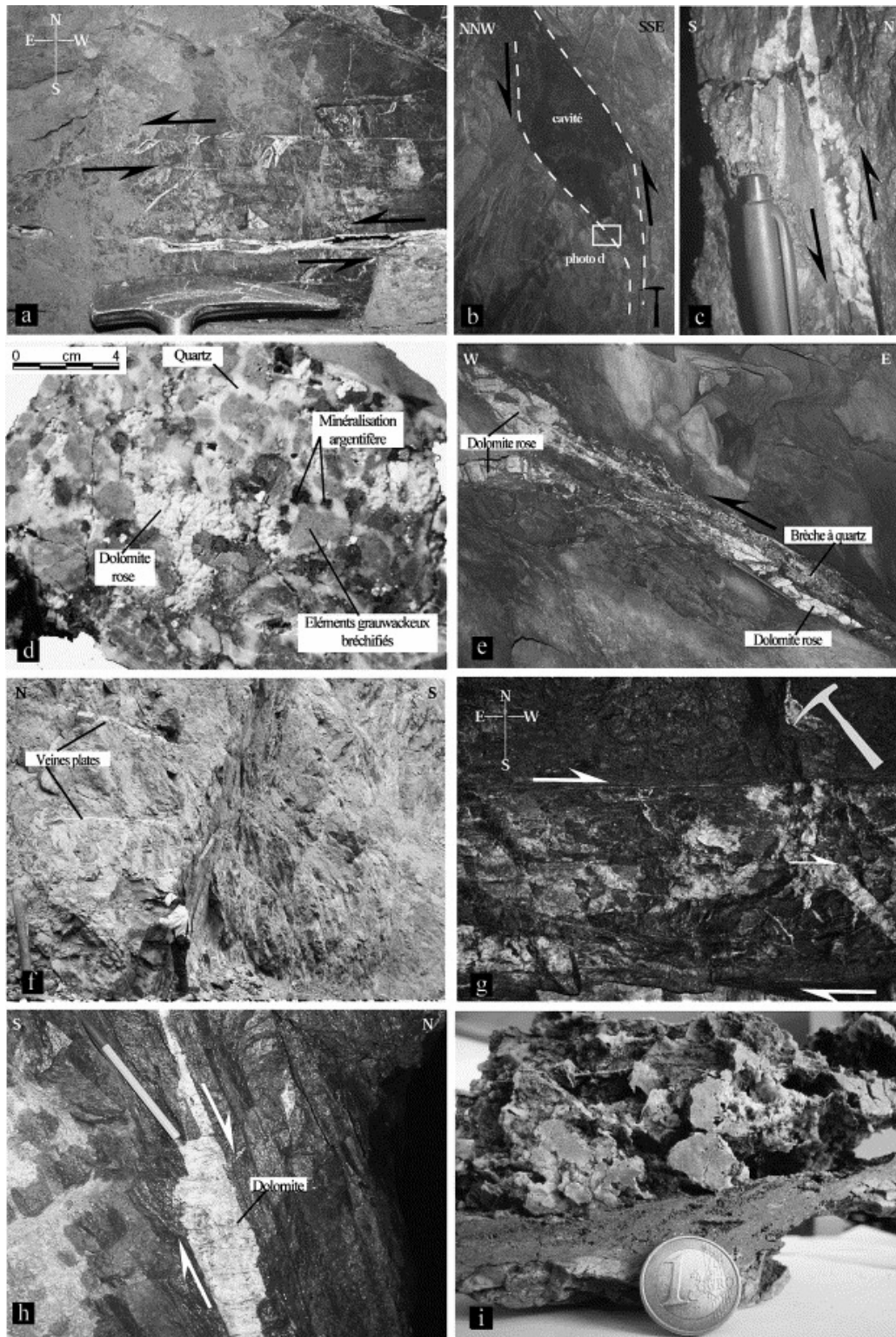
Fig. 4. (a) Vue en couronne des structures du stade 1. Les pull-aparts et les fentes de tension à remplissage géodique de quartz montrent une cinématique dextre, structure F 0 nord, Imiter I. (b) Structures en pull-apart de la F 0 sud, fortement affectées par le stade d'altération entraînant la dissolution du remplissage primaire et la formation d'une cavité (stade 1). L'ouverture de la structure répond à une cinématique chevauchante à vergence nord-ouest-NNW. (c) Pull-apart à remplissage de quartz et boxwork de dolomite rose du stade 1, montrant un cisaillement inverse vers le sud, structure R 6 , Imiter II. (d) Brèche à ciment de quartz, puis dolomite rose altérée du stade 1 et minéralisation argentifère (galène, amalgame Ag-Hg, cuivre gris), rencontrée dans les structures en pull-apart de la structure F 0 sud, Imiter I. Voir la localisation sur la Fig. 4b. (e) Structure plate à remplissage de quartz bréchique puis dolomite rose contrôlée par un jeu chevauchant à vergence ouest-NW, base de la structure
